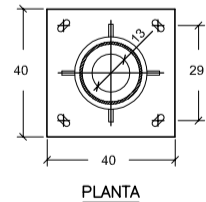
PLANTA COLUMNA
