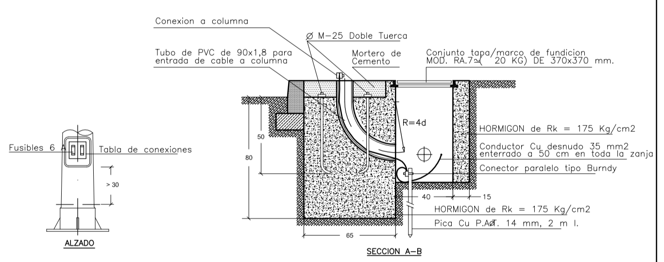
SECCION A-B
