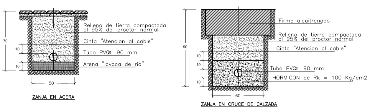
DETALLE DE CANALIZACIONES
