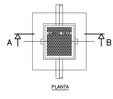
DETALLE DE ARQUETA
