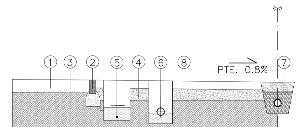
SECCIÓN ACERADO E 1/100
