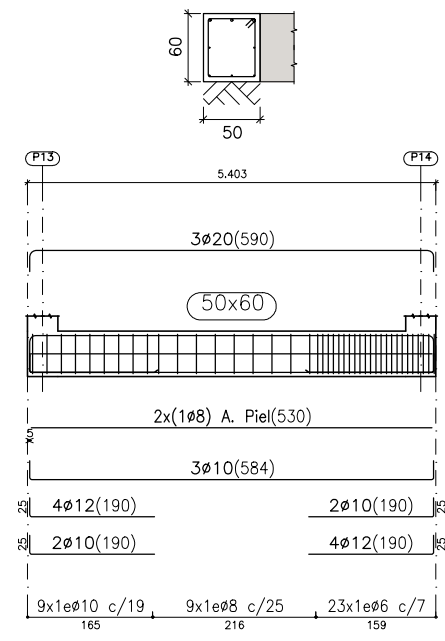
Pórtico 4 Ver arranques en el despiece de pilares o alzado de muros
