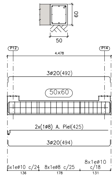
Pórtico 3 Ver arranques en el despiece de pilares o alzado de muros
