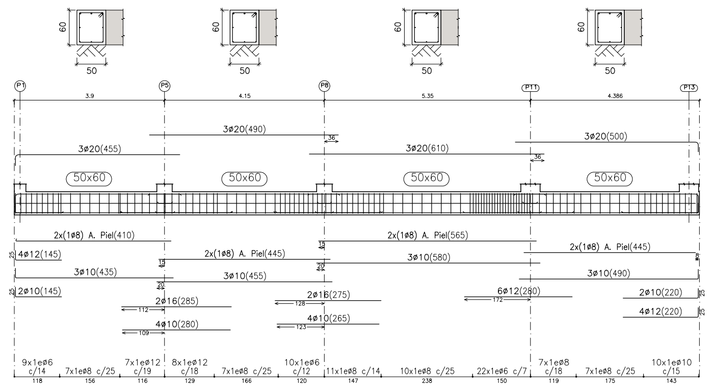
Pórtico 5 Ver arranques en el despiece de pilares o alzado de muros
