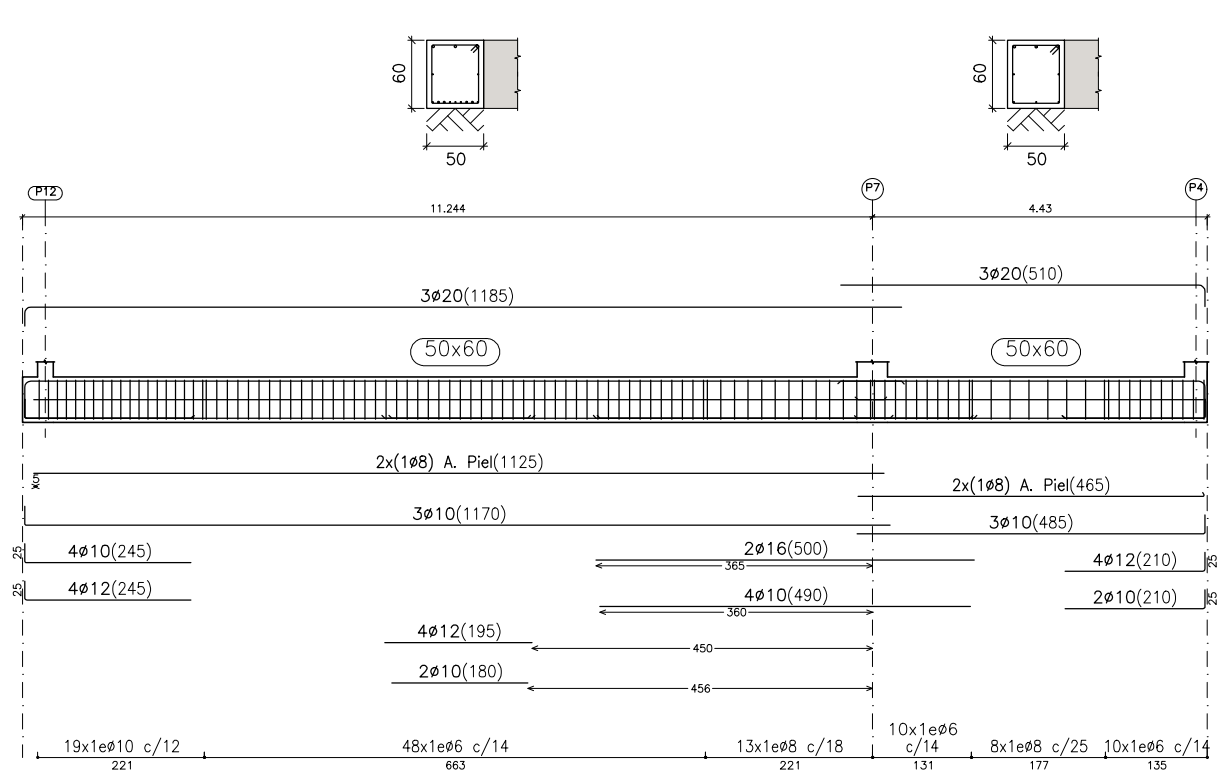
Pórtico 2 Ver arranques en el despiece de pilares o alzado de muros
