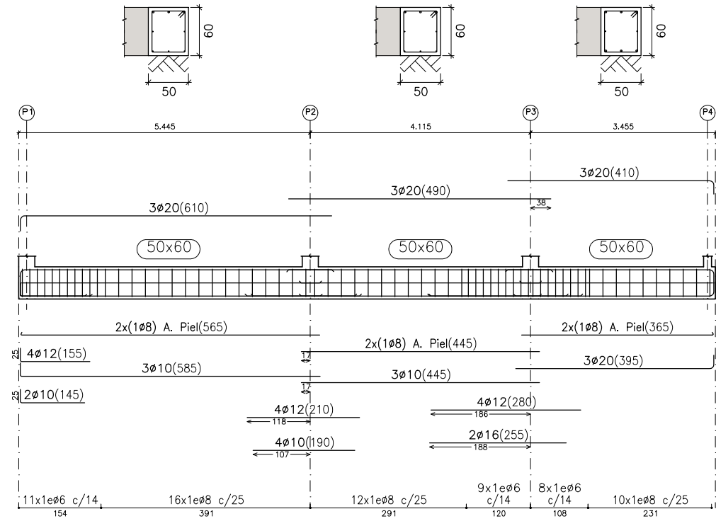
Pórtico 1 Ver arranques en el despiece de pilares o alzado de muros
