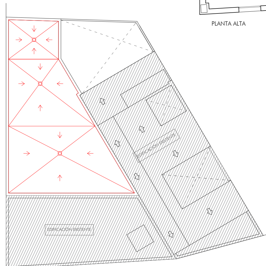
PLANTA CUBIERTA
